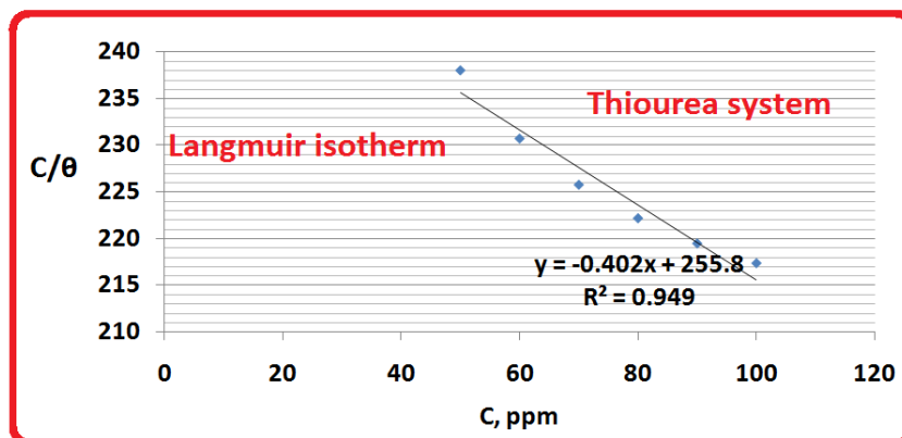
Figure 7. Langmuir adsorption isotherm for Thiourea (TU) system Slika 7. Langmuirova adsorpciona izoterma za sistem Thiourea (TU)
