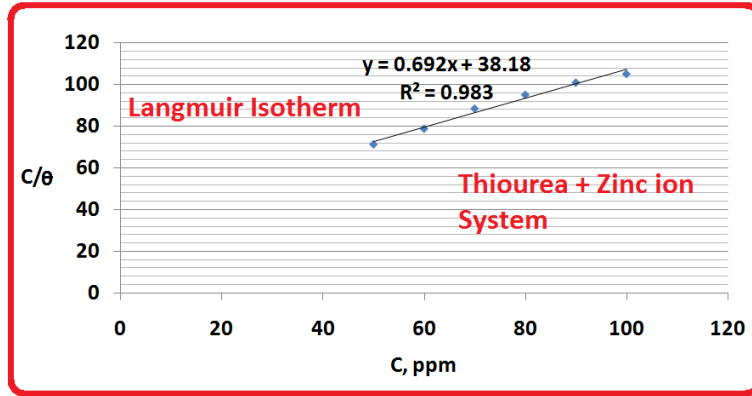
Figure 8. Langmuir adsorption isotherm for Thiourea (TU) - Zn 2+ system Slika 8. Langmuirova adsorpciona izoterma za sistem Thiourea (TU) - Zn 2+
