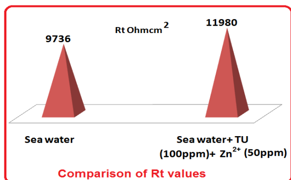
Figure 13. Comparison of Rt values Slika 13. Poređenje vrednosti Rt
