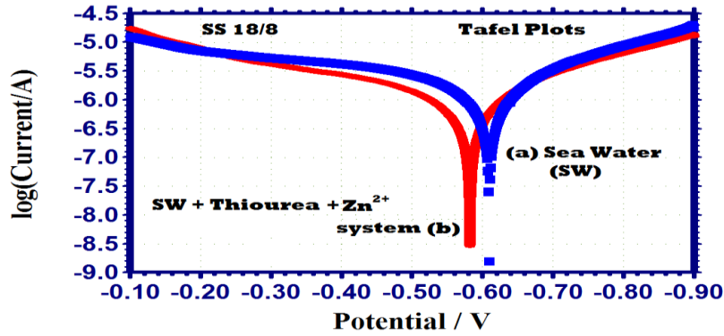
Figure 9. Tafel plots of various test solutions Slika 9. Tafelov prikaz različnih rešenja ispitivanja
