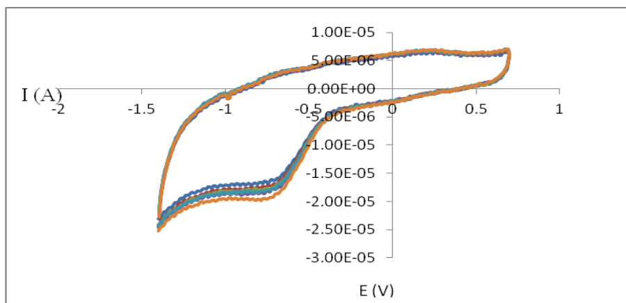
Slika 2. Ciklični voltamogram GC elektrode u prisustvu različite koncentracije aktivne supstance perindopрила u fosfatnom puferu: — 0 mg/mL; — 1,5987 × 10 -4 mg/mL; — 3,1948 × 10 -4 mg/mL; — 4,7885 × 10 -4 mg/mL; — 6,3795 × 10 -4 mg/mL; — 7,9681 × 10 -4 mg/mL
