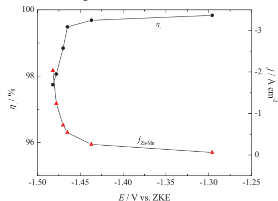
Slika 2 - Iskorišćenje struje i polarizaciona kriva taloženja Zn-Mn legure ( j_{Zn-Mn} ) u sulfatnom rastvoru
