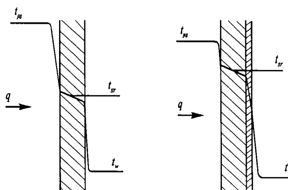
Slika 1 - Uticaj kamenca na temperaturu kotlovske materijala [4]
