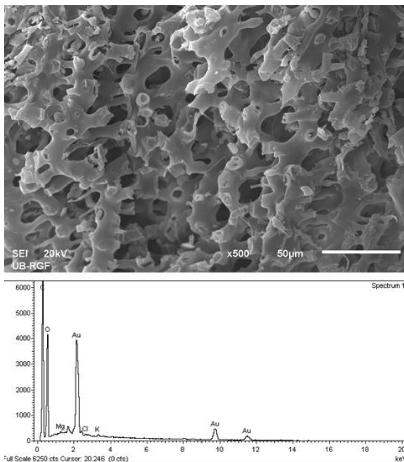
Slika 2 - SEM mikrografija i EDX spektar OK
