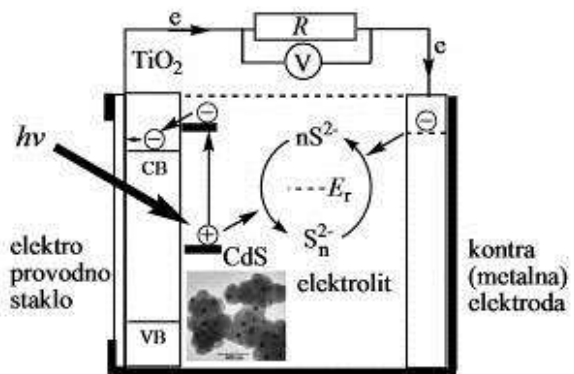
Slika 9 - Shematski prikaz funkcionisanja solarna ćelija aktivirana kvantnim česticama (QDSSC)
