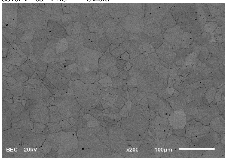
Slika 1 - Izgled snimka urađenog uređajem SEM, sa uvećanjem x200 ; Elementi obrade: t=200^\circ C , \tau = 30 min, 169.80HV0.25 . Struktura ravnoosnih kristala, dobijenih rekristalizacionim žerenjem, sa velikom količinom dvojnika žarenja dobijenih starenjem
