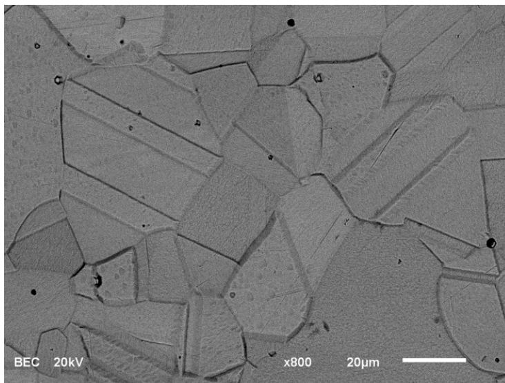
Slika 3 - Izgled dela slike 1, snimak SEM-a, sa uvećanjem x800. Izrazito istaknuti dvojnici žarenja
