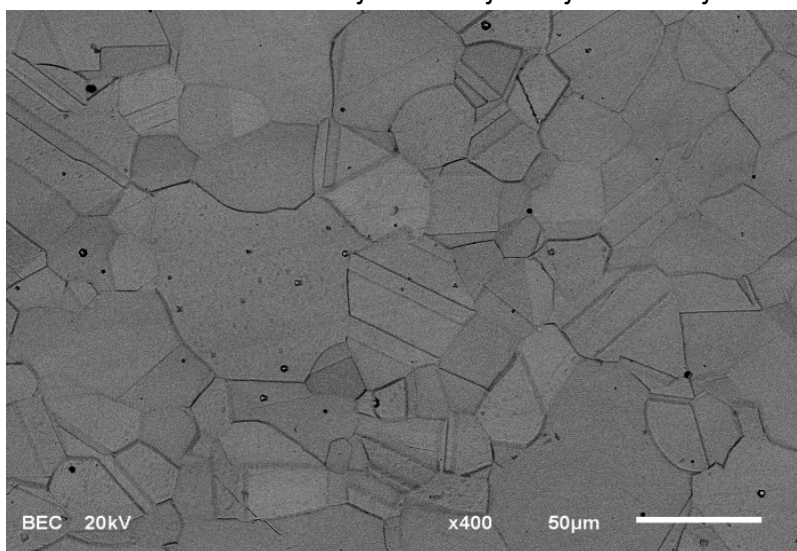
Slika 2 - Izgled snimka SEM sa slike 1, sa uvećanjem x400 . Ističe se pojava dvojnika žarenja u strukturi legure
