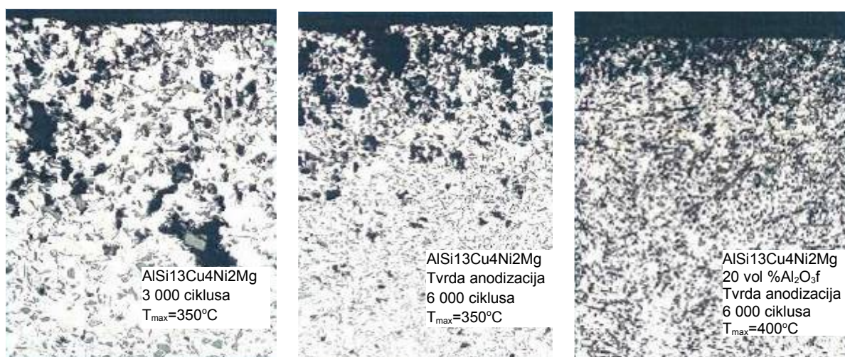
Slika 2 – Ispitivanje anodnog sloja klipova od legure AlSi13Cu4Ni2Mg[1]
