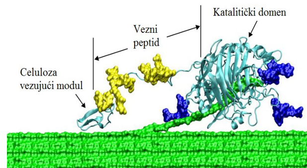
Slika 3 - Građa i mehanizam delovanja celobihidrolaze [25]
