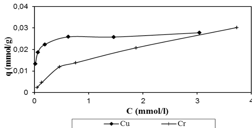
Slika 1 - Adsorpcione izoterme za adsorpciju jona bakra i hroma (VI) tehničkom celulozom
