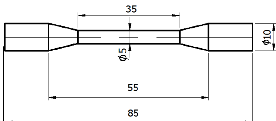
Slika 5 - Epruveta za ispitivanje
