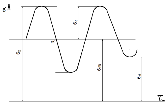
Slika 3 - Karakteristične veličine u dijagramu napon – vreme
