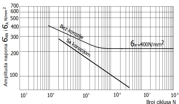
Slika 10 - Dijagram zamaranja za čelik Č.0545 pri dejstvu korozije (σ sr = 400N/mm 2 )
