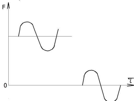
Slika 2 - Karakteristični slučajevi jednosmerno promenljivog i naizmenično promenljivog opterećenja u dijagramu opterećenje – vreme
