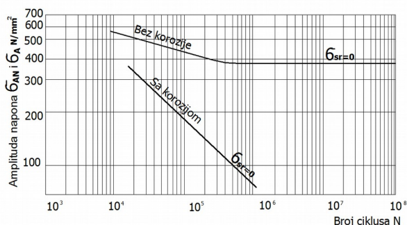
Slika 9 - Dijagram zamaranja za čelik Č.0545 pri dejstvu korozije (σ sr = 0)
