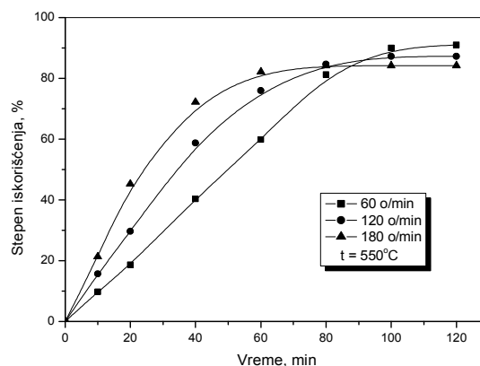
Slika 7 - Zavisnost stepena iskorišćenja olova od brzine mešanja
