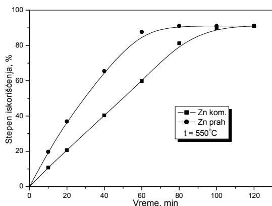
Slika 6 - Zavisnost stepena iskorišćenja olova od oblika korišćenog cinka
