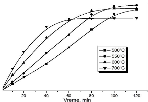
Slika 5 - Zavisnost stepena iskorišćenja olova od temperature i vremena postupkom cinkotermije
