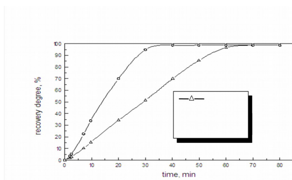
Slika 4 - Zavisnost stepena iskorišćenja olova od vremena i oblika korišćenog aluminijuma
